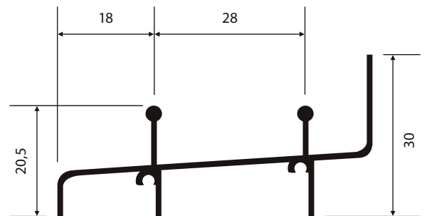
MP-370 0,565 Kg/m
