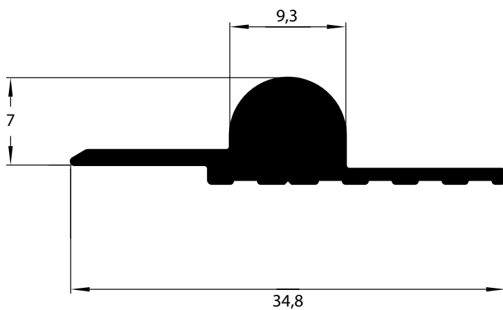
NI-2125 0,269 Kg/m
