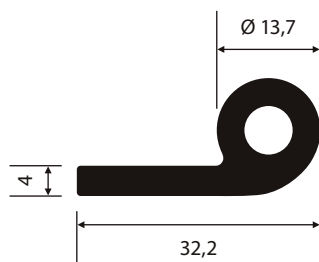
NI-075 0,578 Kg/m
