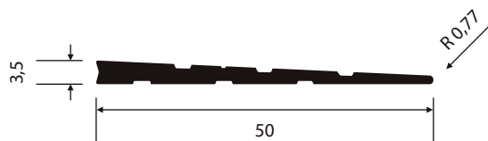
CL-011 0,319 Kg/m
