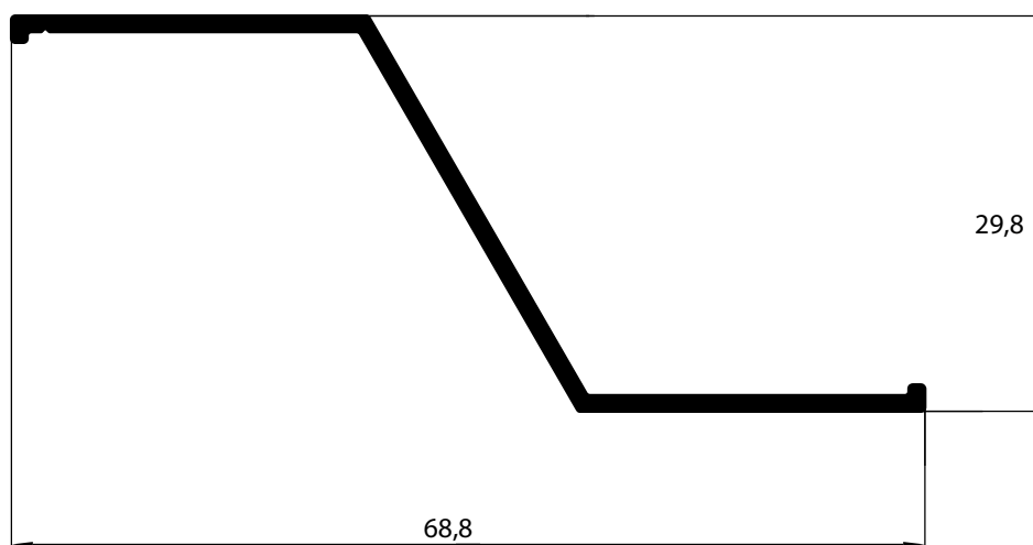
VZ060A 0,282 Kg/m
