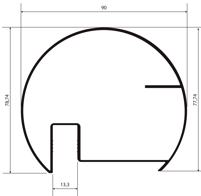
NI-1103 1,385 Kg/m
