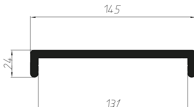
NI-2132 3,555 Kg/m
