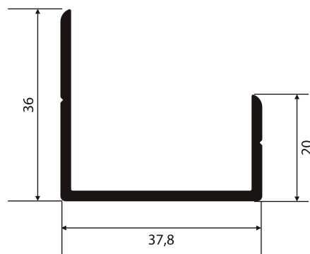
NI-1022 0,478 Kg/m
