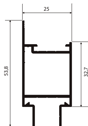
SU-192 0,507 Kg/m
