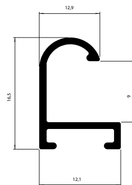
NI-541 0,115 Kg/m
