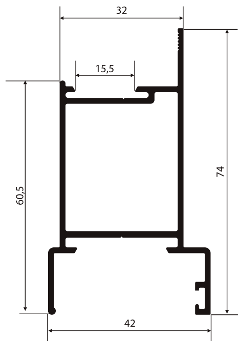
NI-515 0,920 Kg/m
