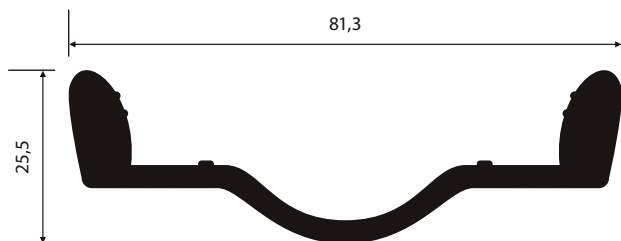
NI-378 1,324 Kg/m
