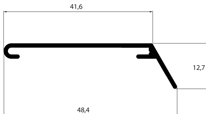
NI-1373 0,215 Kg/m
