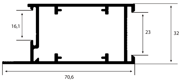
LG-043 0,834 Kg/m
