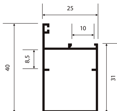
P-140 0,436 Kg/m
