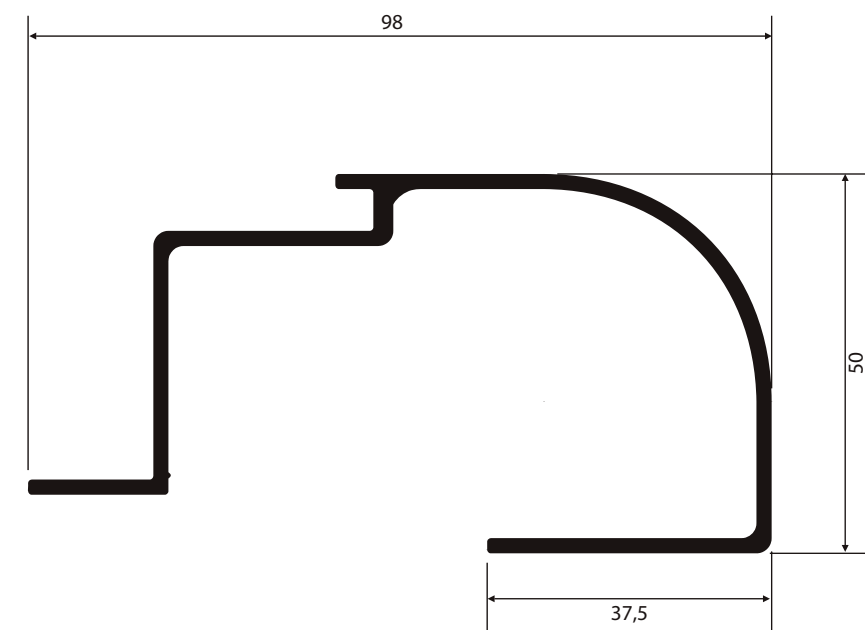
NI-363 1,177 Kg/m
