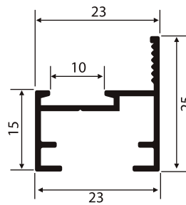
NI-760 0,249 Kg/m
