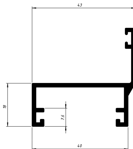
Y-181 0,535 Kg/m
