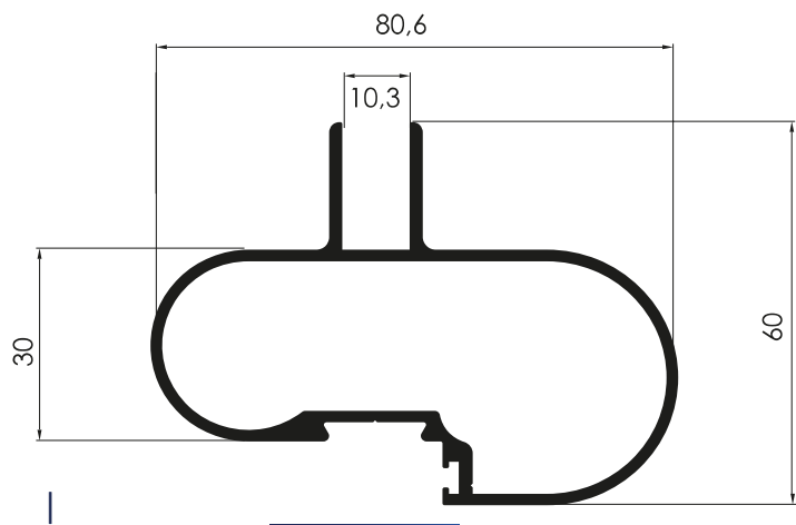
DV-300 1,416 Kg/m
