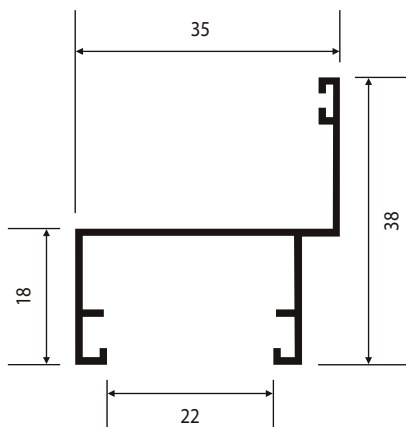
Y-140 0,386 Kg/m
