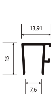
NI-119 0,134 Kg/m
