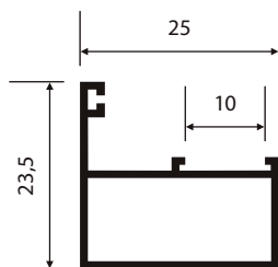
P-147 0,351 Kg/m
