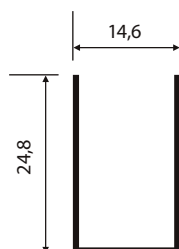
U-555A 0,168 Kg/m
