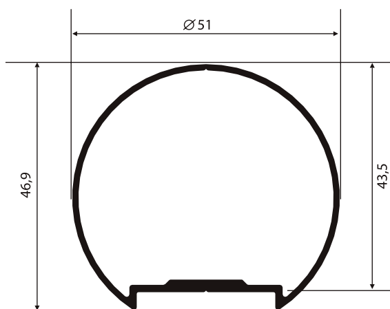
NI-742 0,583 Kg/m
