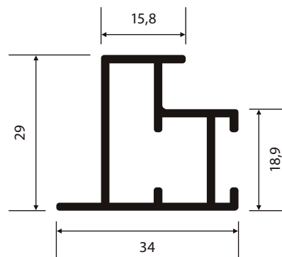
NI-162 0,483 Kg/m
