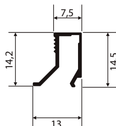
BG-202 0,106 Kg/m
