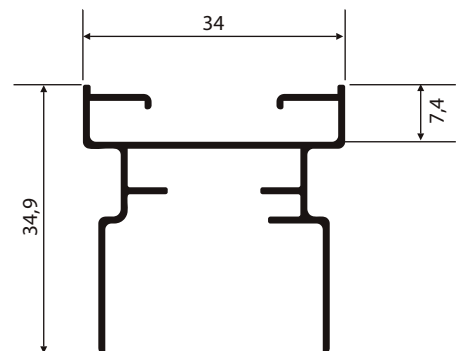
NI-130 0,341 Kg/m
