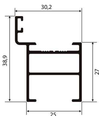
P-412A 0,439 Kg/m
