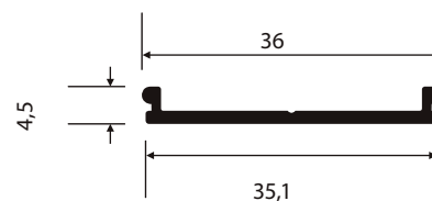
U-495 0,170 Kg/m
