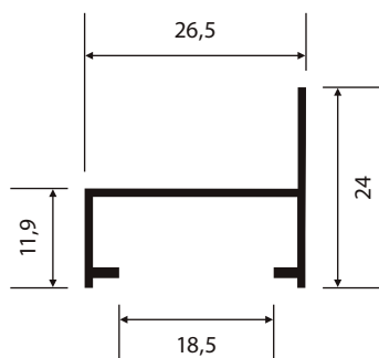
CM-063 0,180 Kg/m
