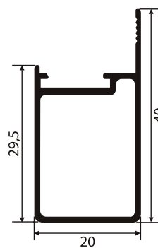
MP-300 0,334 Kg/m
