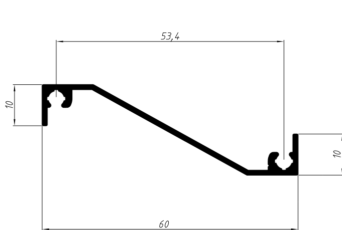
Z073 0,331 Kg/m
