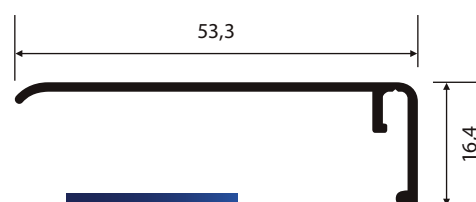
NI-283 0,220 Kg/m
