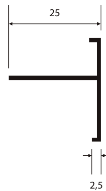
T-095 0,190 Kg/m
