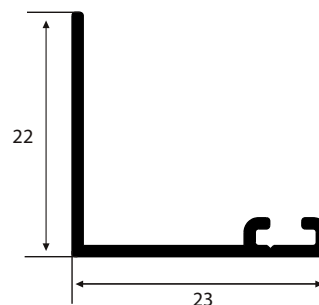
NI-1315 0,137 Kg/m
