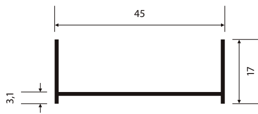
U-399 0,228 Kg/m
