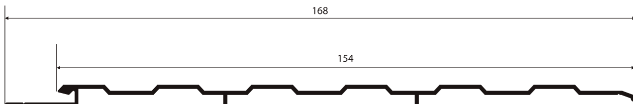
Y-429MA 0,580 Kg/m
