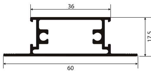
MP-332 0,489 Kg/m
