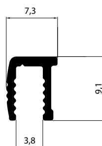
NI-1279 0,072 Kg/m
