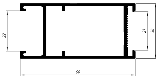
A-144 0,766 Kg/m
