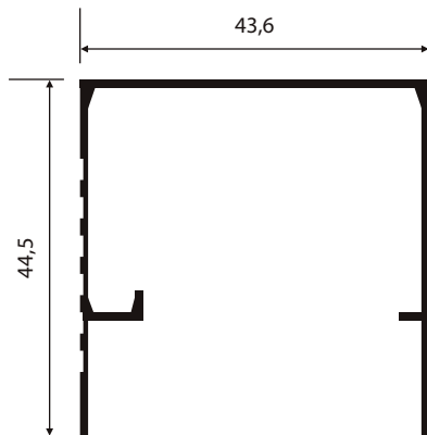
NI-150 0,421 Kg/m
