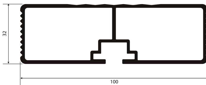
NI-537 1,353 Kg/m
