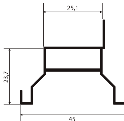
NI-013 0,349 Kg/m
