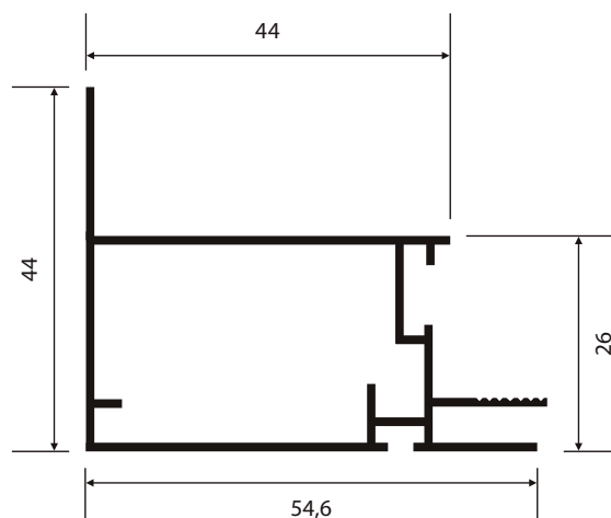
MP-069 0,602 Kg/m
