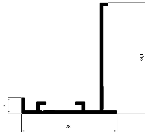
NI-1344 0,224 Kg/m
