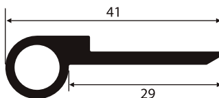
NI-432 0,395 Kg/m
