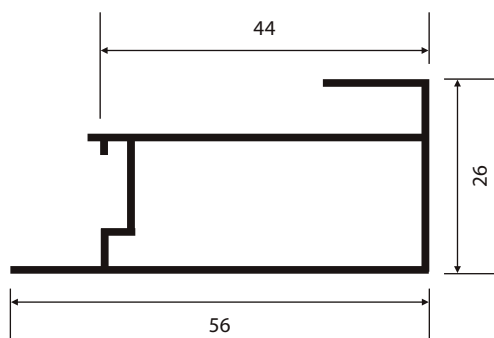
MP-070 0,497 Kg/m
