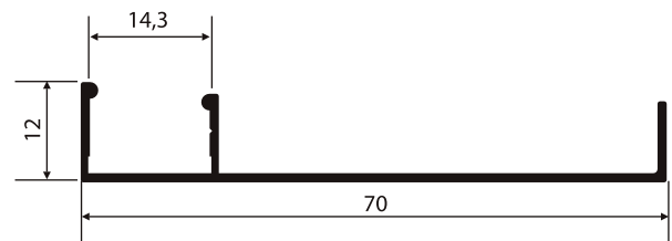
NI-944 0,301 Kg/m
