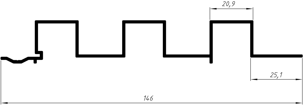
NI-2079 0,858 Kg/m
