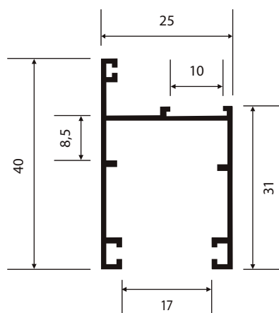
Y-195 0,432 Kg/m
