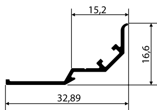
SU-083 0,143 Kg/m
