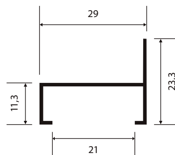
Y-120 0,250 Kg/m
