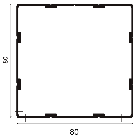
NI-394 1,171 Kg/m
