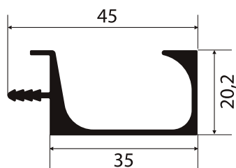
NI-015 0,517 Kg/m
