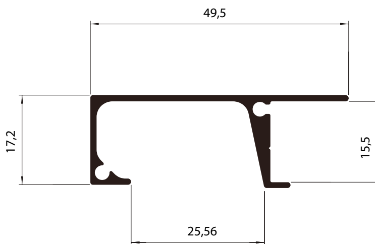
NI-4065 0,372 Kg/m
