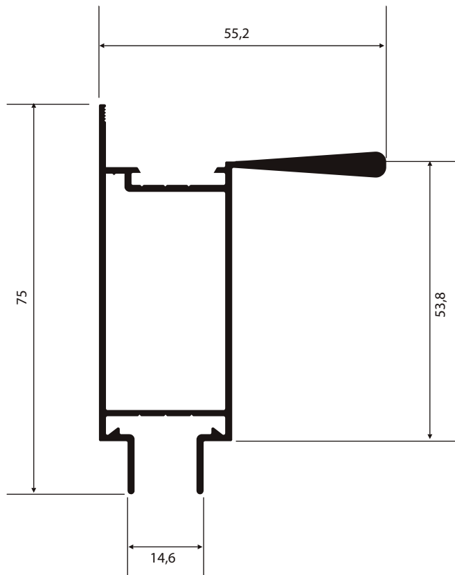
SU-281 0,986 Kg/m
