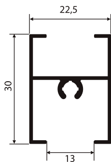
NI-009 0,308 Kg/m
