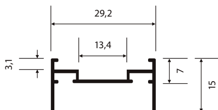
I-105 0,220 Kg/m
