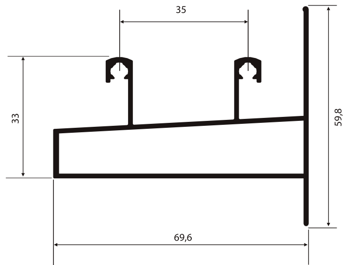
SU-006 0,982 Kg/m
