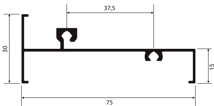
NI-568 0,549 Kg/m
