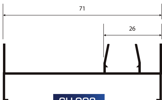
SU-003 0,494 Kg/m
