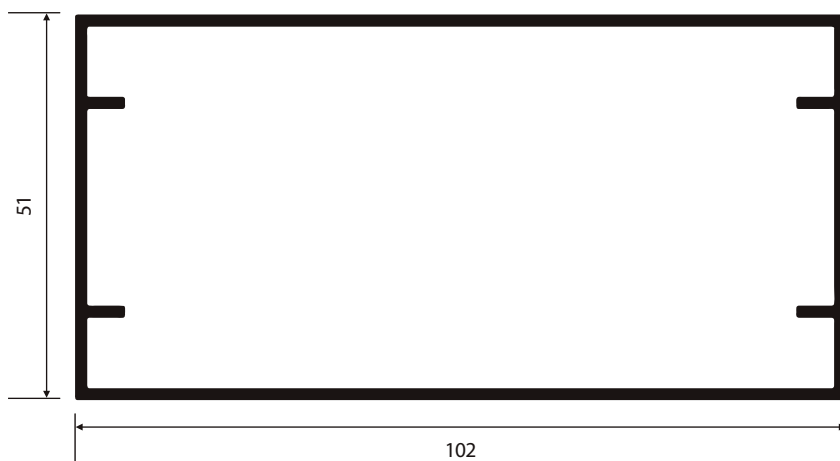
NI-1010 0,571 Kg/m
