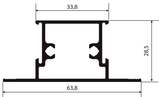
NI-516 0,742 Kg/m
