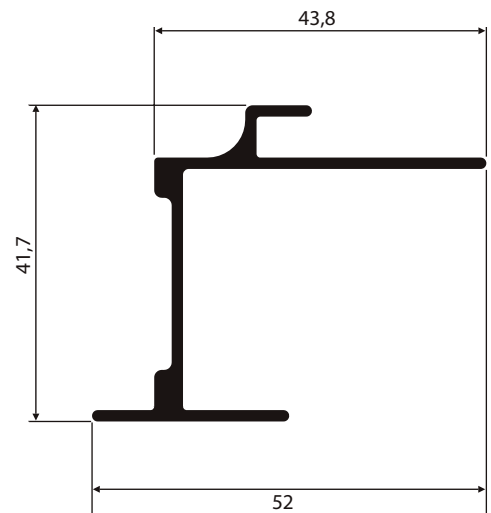
NI-486 0,539 Kg/m
