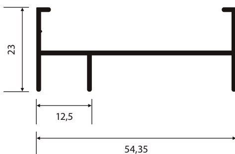
LE-1616 0,396 Kg/m
