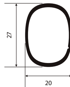
NI-232 0,296 Kg/m
