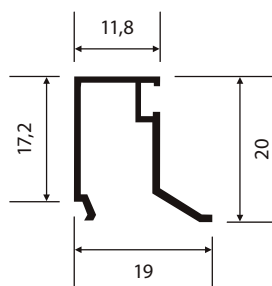
U-1027 0,162 Kg/m
