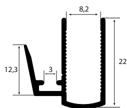
NI-2156 0,651 Kg/m
