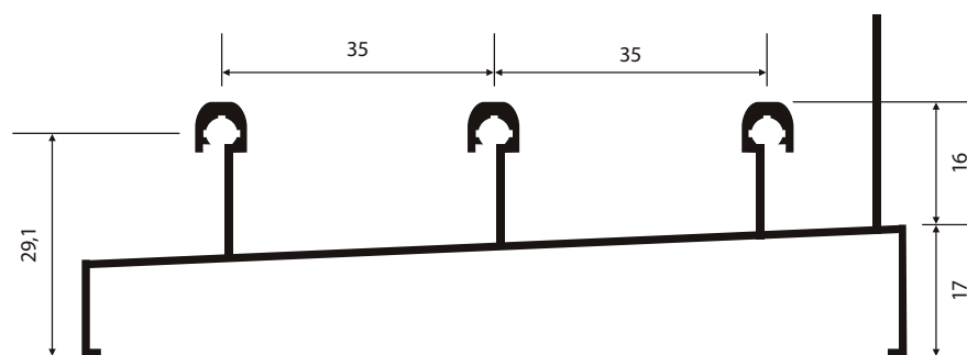
SU-011 0,973 Kg/m
