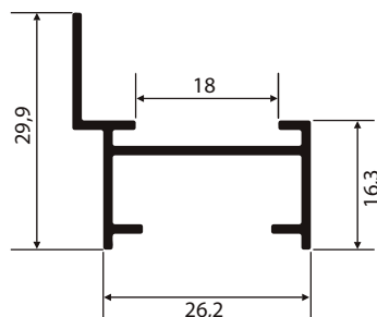
SU-071 0,283 Kg/m
