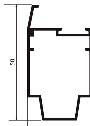
NI-858 0,468 Kg/m
