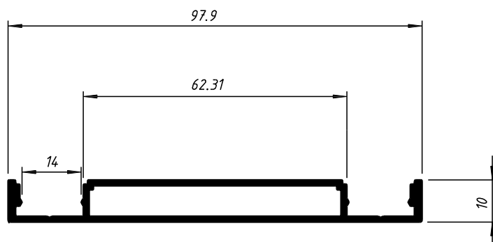
NI-1002 0,779 Kg/m
