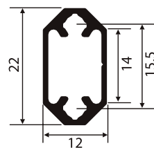
NI-761 0,229 Kg/m
