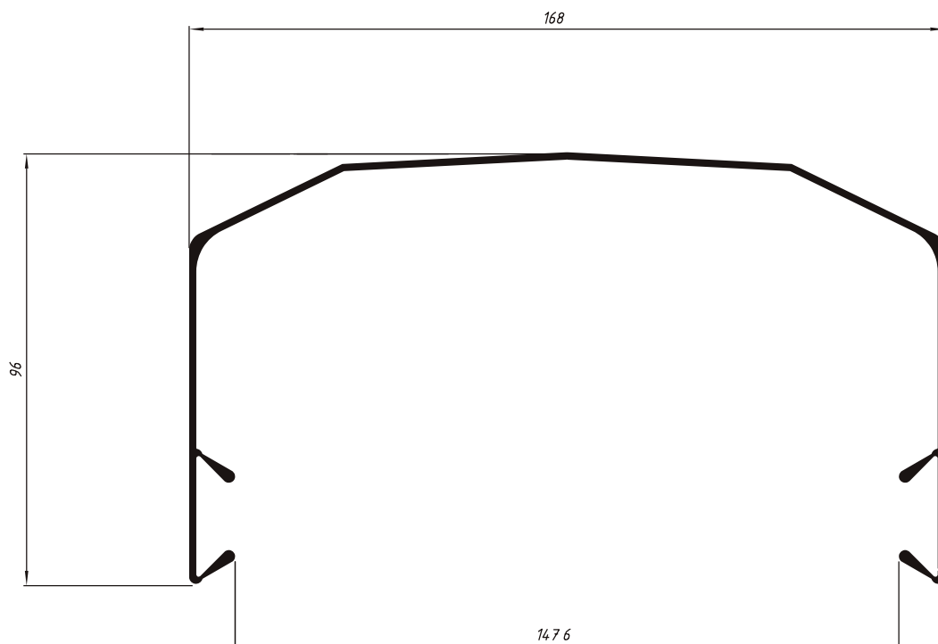
NI-1504 1,646 Kg/m
