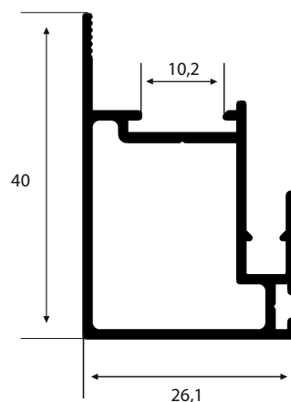
MP-302MA 0,375 Kg/m
