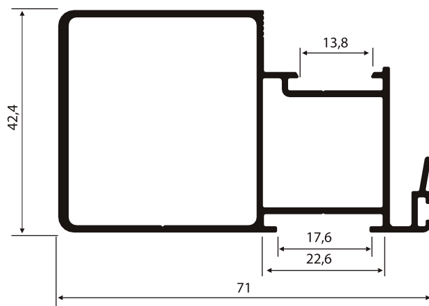
SU-049 1,042 Kg/m
