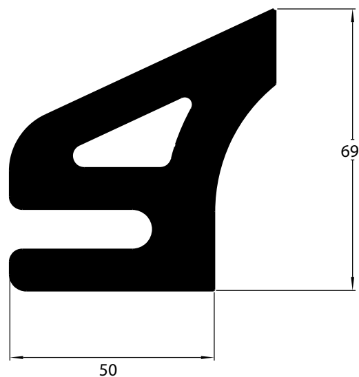
NI-2197 6,064Kg/m
