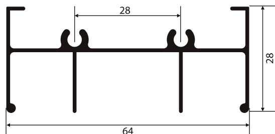
MP-357 0,558 Kg/m
