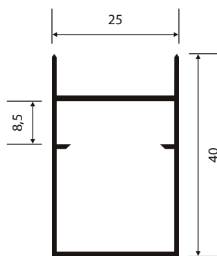
A-055 0,434 Kg/m
