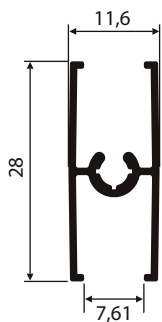
NI-651 0,211 Kg/m
