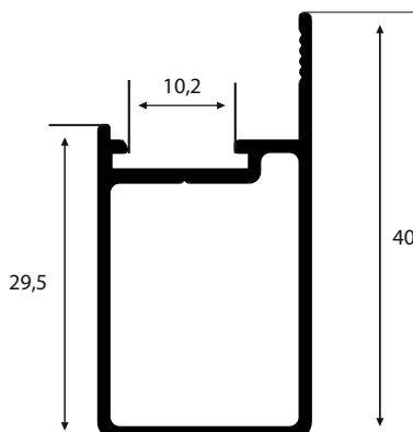
MP-300MA 0,307 Kg/m
