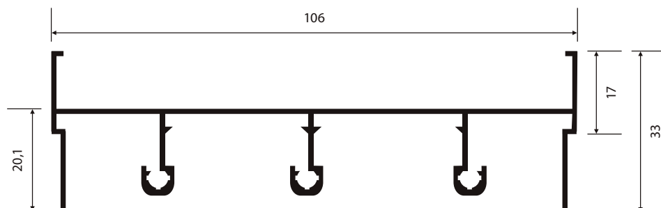
SU-010 0,960 Kg/m
