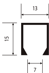
U-425 0,155 Kg/m
