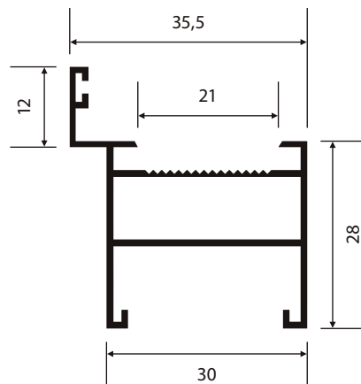
P-273 0,563 Kg/m
