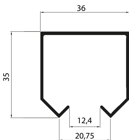
NI-3039 0,406 Kg/m
