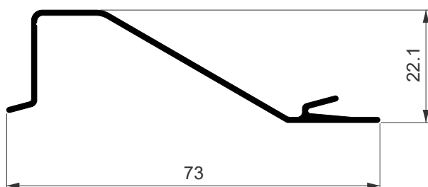
NI-2297 0,305 Kg/m
