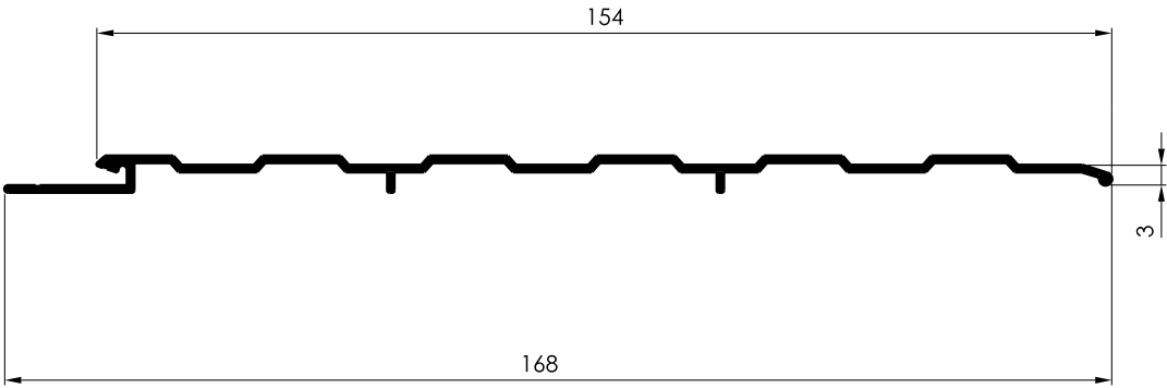
Y-429L 0,526 Kg/m
