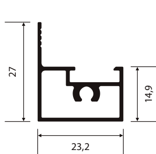
25-301 0,306 Kg/m
