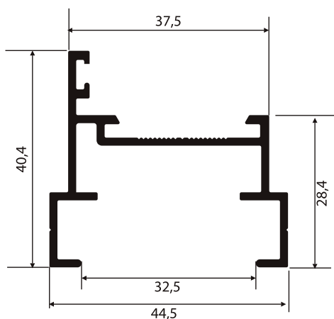
NI-517 0,582 Kg/m
