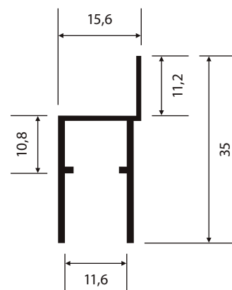
Y-106 0,245 Kg/m
