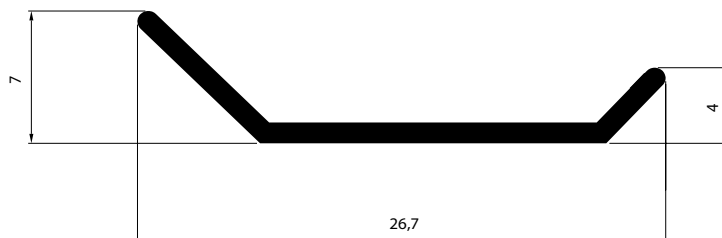
NI-1346 0,089 Kg/m
