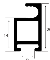
A-058 0,220 Kg/m
