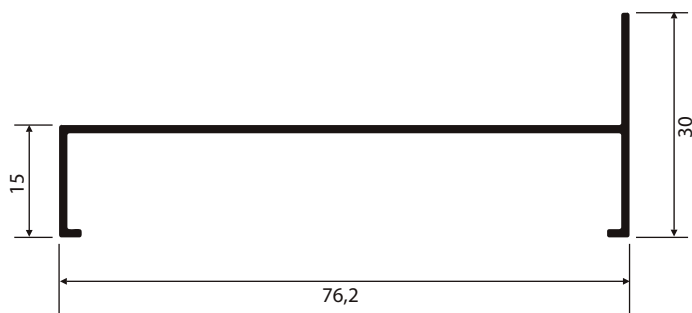
NI-567 0,366 Kg/m
