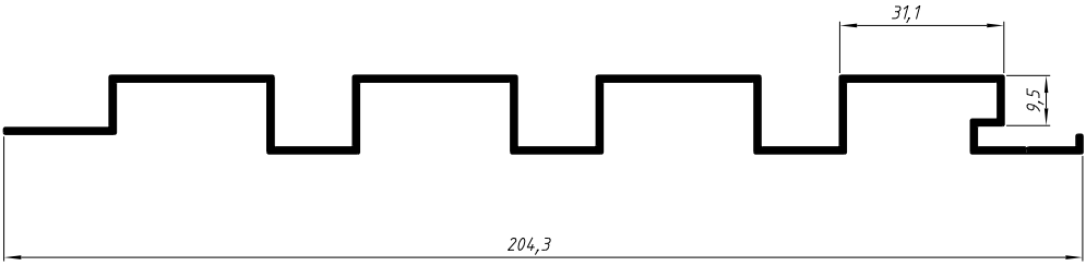
NI-2078 1,046 Kg/m
