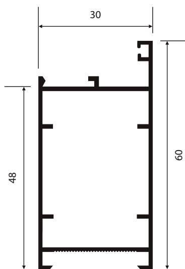
P-270 0,793 Kg/m
