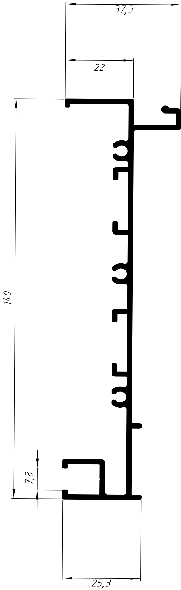
MN-001 1,179 Kg/m
