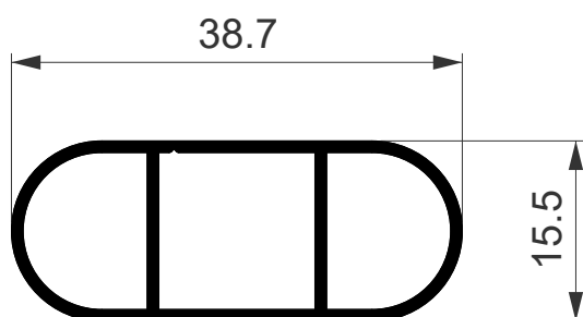
NI-2262 0,322 Kg/m
