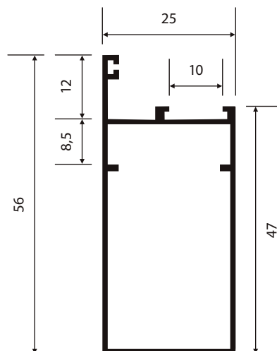
P-318 0,553 Kg/m
