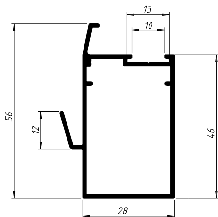
NI-856 0,549 Kg/m
