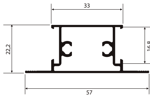
SU-227 0,504 Kg/m
