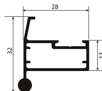
NI-946 0,413 Kg/m
