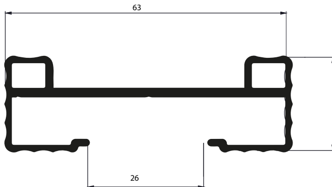
NI-1209 0,680 Kg/m
