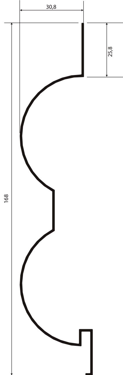
LB-070 0,763 Kg/m
