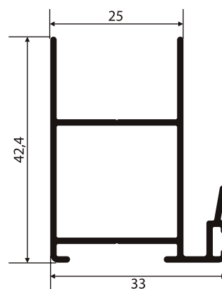
SU-070 0,518 Kg/m
