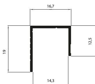
NI-1727 0,145 Kg/m
