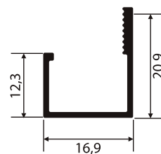
NI-1105 0,165 Kg/m
