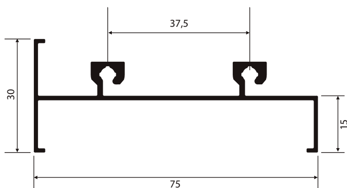
NI-569 0,613 Kg/m
