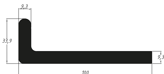
NI-2155 3,115 Kg/m
