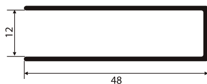
NI-841 0,350 Kg/m
