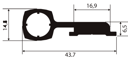
NI-690 0,623 Kg/m
