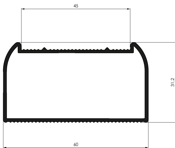
NI-1345 0,627 Kg/m
