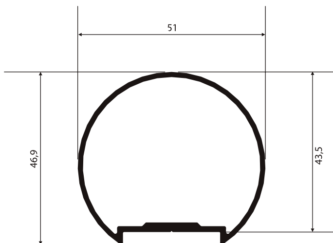
NI-680 0,668 Kg/m
