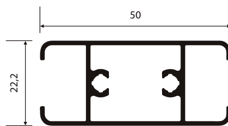
SU-188 0,591 Kg/m
