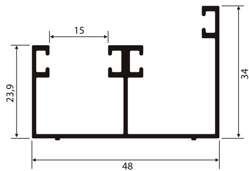
NI-543 0,534 Kg/m
