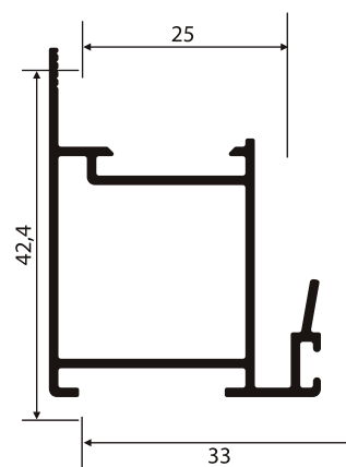
SU-041 0,508 Kg/m
