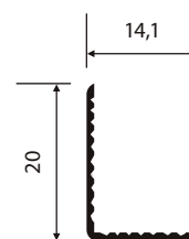
U-1109 0,163 Kg/m
