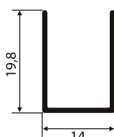
NI-717 0,139 Kg/m
