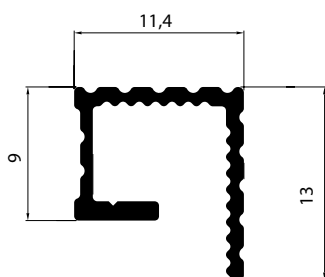
NI-1276 0,097 Kg/m
