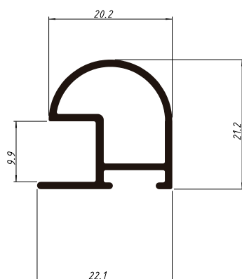
NI-604 0,265 Kg/m
