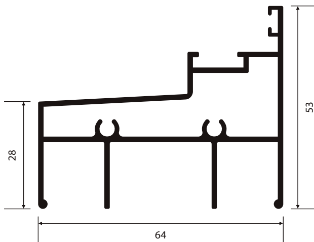
MP-361 1,074 Kg/m
