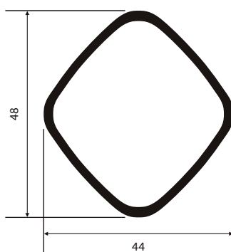
XKS-04 0,766 Kg/m
