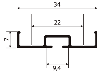
NI-126 0,163 Kg/m
