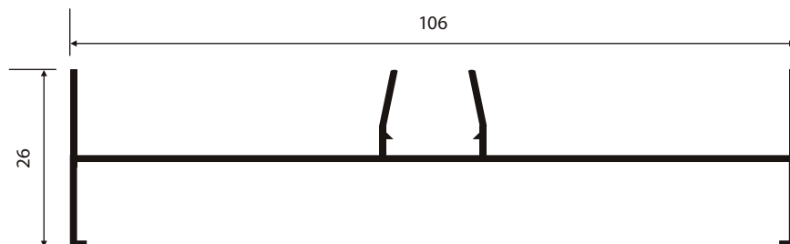
SU-014 0,648 Kg/m
