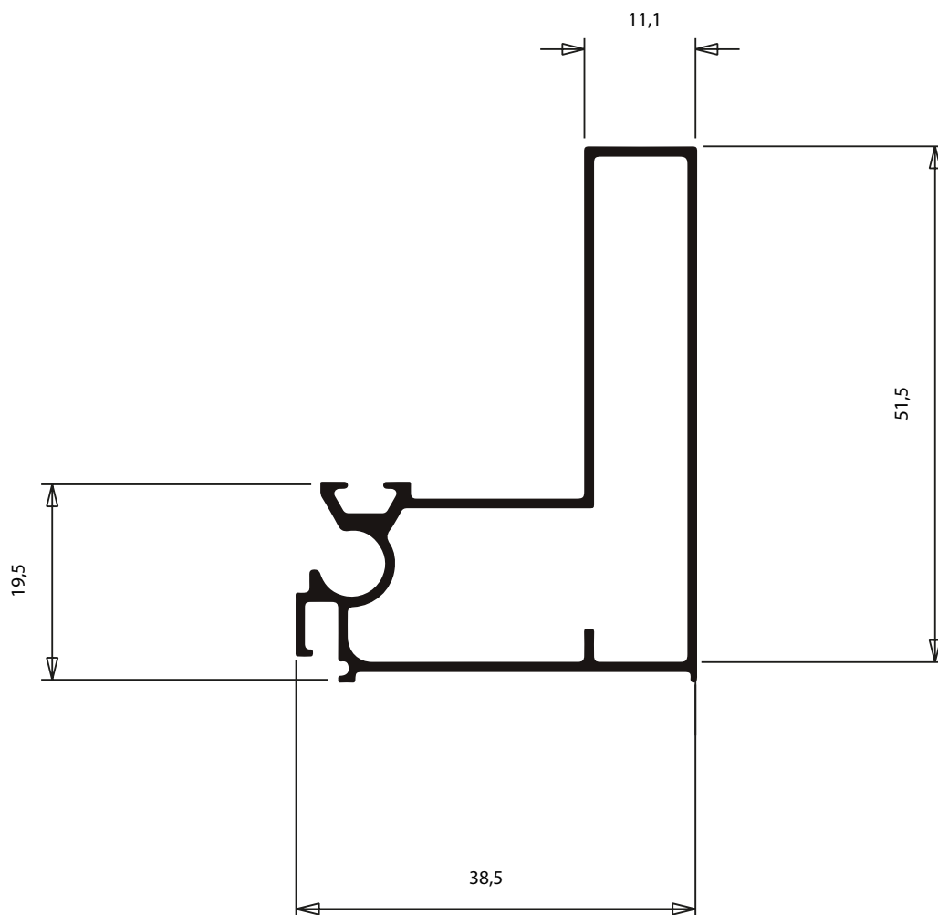
FA-245 0,690 Kg/m
