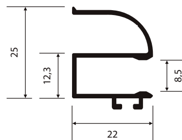
NI-282 0,269 Kg/m
