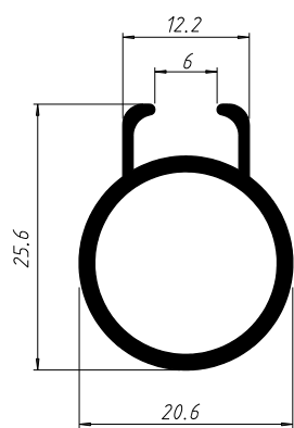
NI-099 0,291 Kg/m
