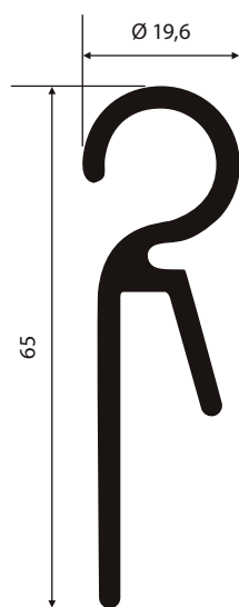
NI-060 0,888 Kg/m
