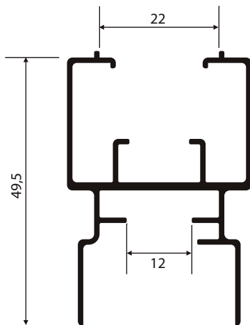
NI-129 0,557 Kg/m
