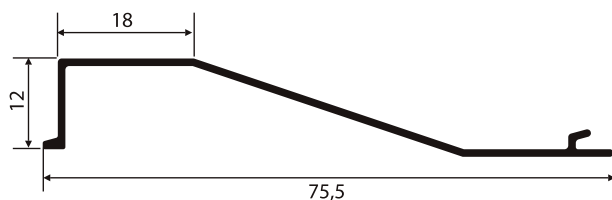
Z-169A 0,252 Kg/m
